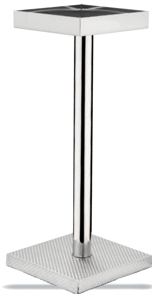
mm. 1,2 FASHION Colonna portasecchiello spumante Wine cooler stand Pied pour seau à champagne Weinkühlerständer Columna porta cubo champany H cm. 61,5 H 24 1/5"
